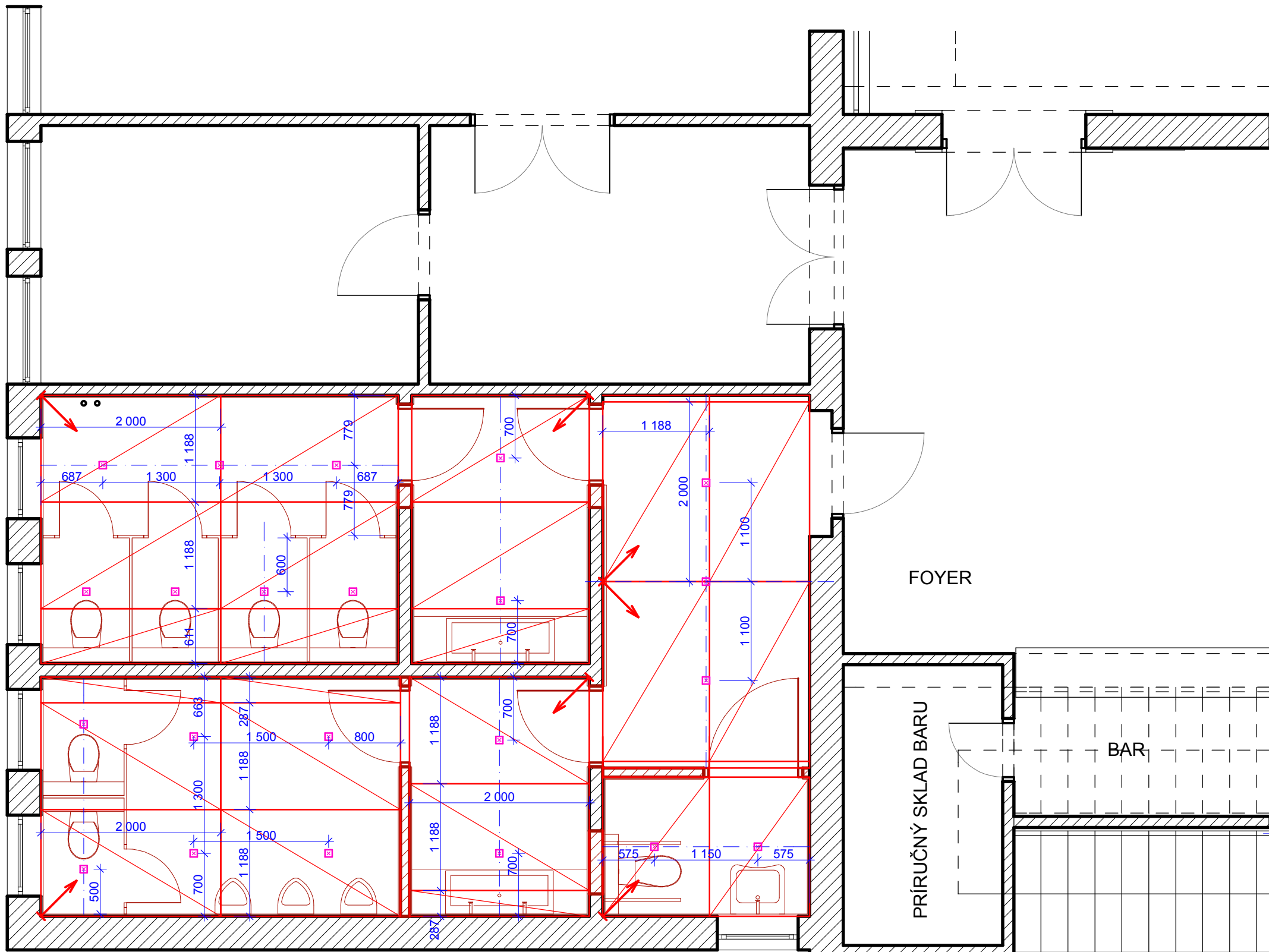
PÔDORYS - PODHLAD
